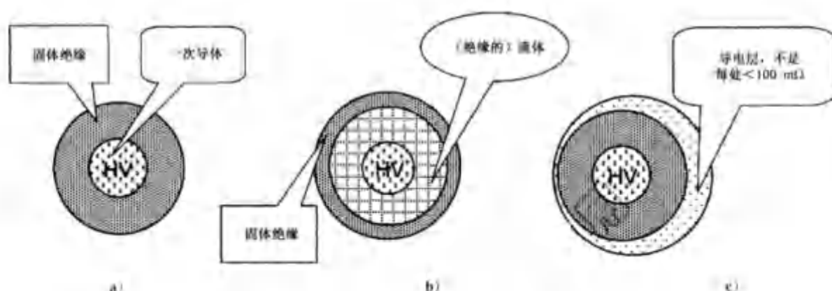
图 C.1 防护等级 PA 的可能设计
