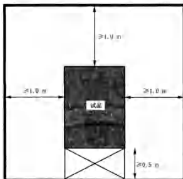
图 E.2 气候试验室
