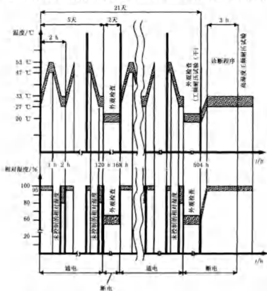
图 E.3 1级老化试验
