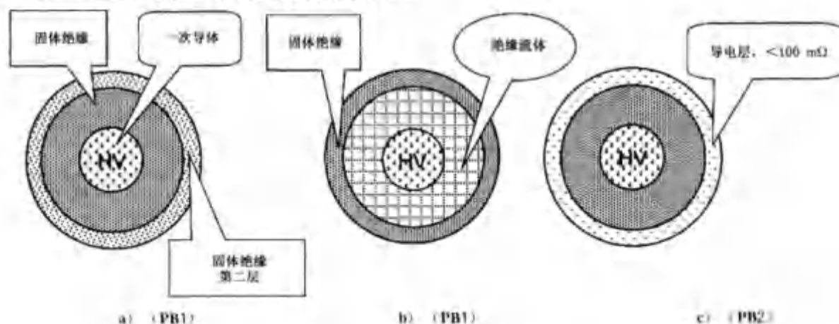
图 C.2 防护等级 PB 的可能设计
