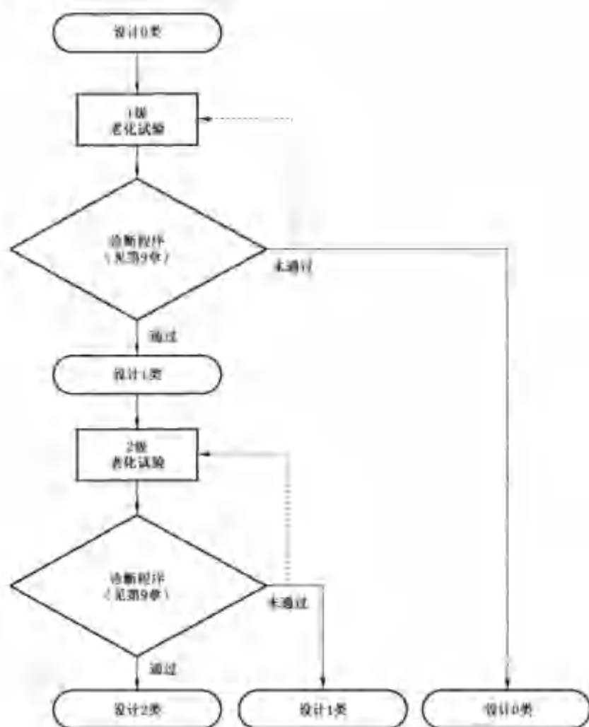
图 E.1 分类程序的流程图
